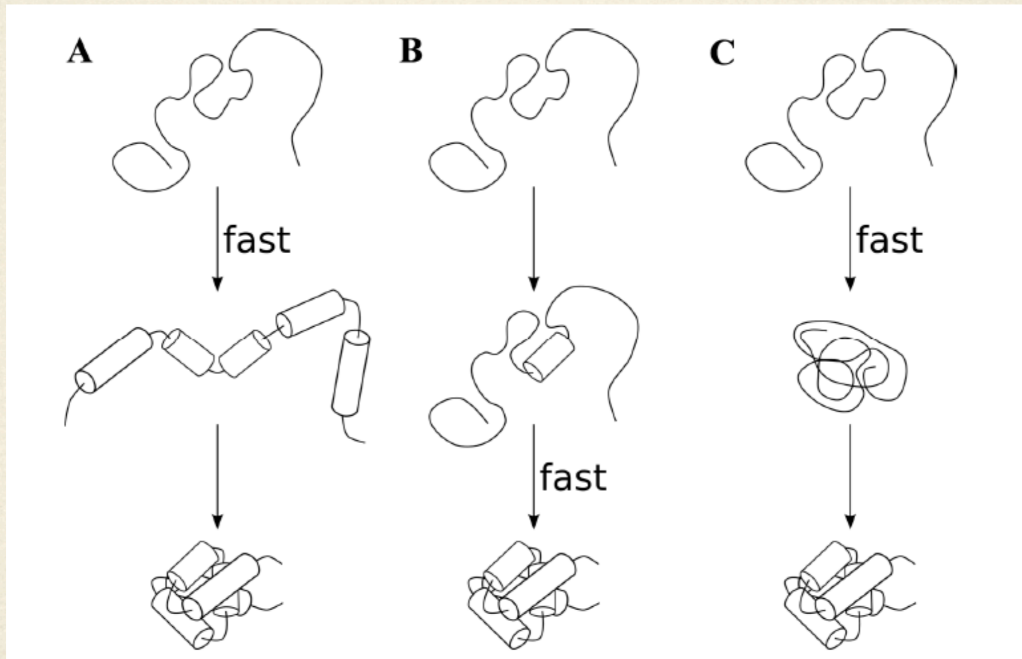
model dyfuzyjno-kolizyjny
