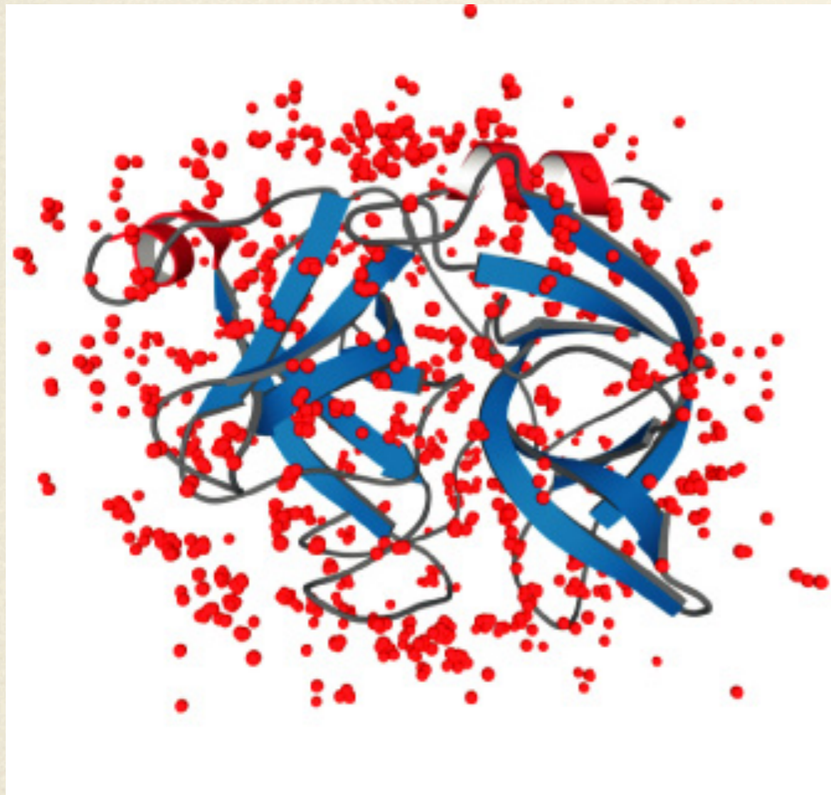
Pierwsza powłoka hydratacyjna elastazy
