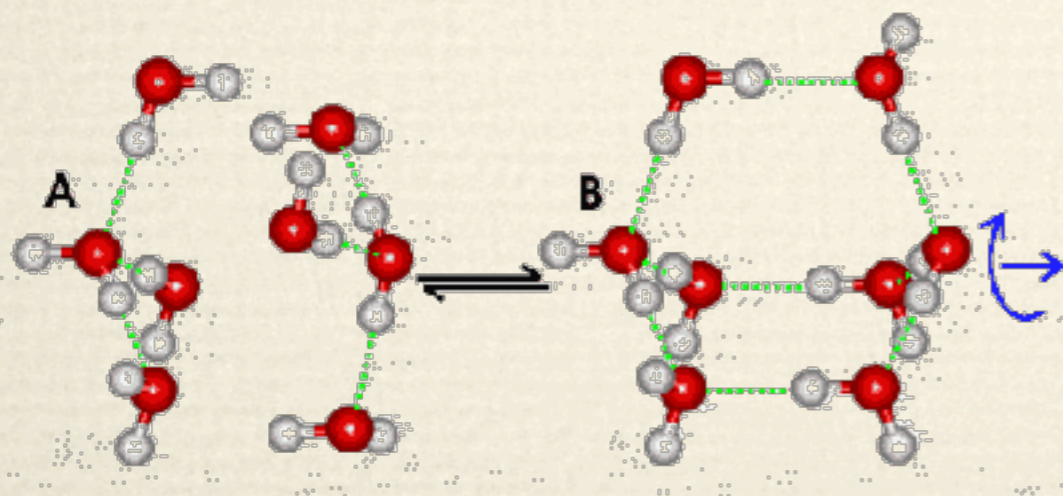
Dwa wodne tetramery tworzące klaster oktamerowy
